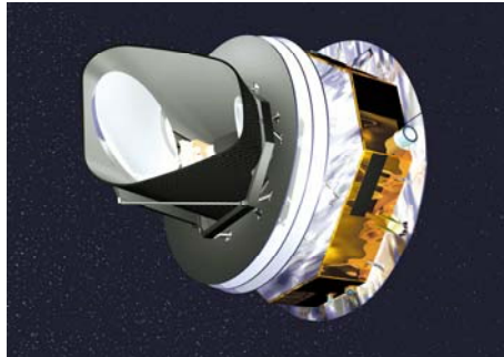
Planck © ESA
